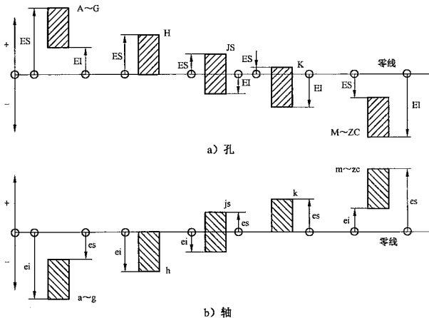
图 1 上极限偏差和下极限偏差
